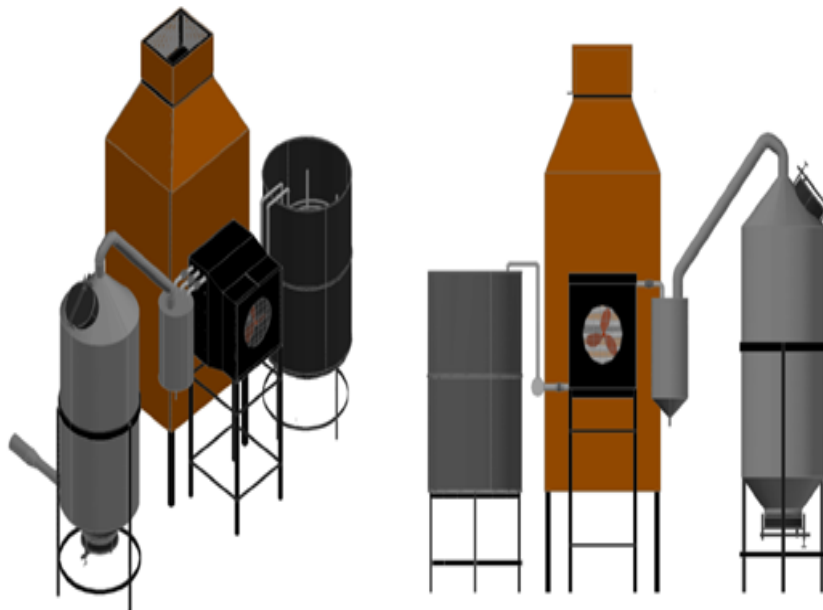
Gambar 4. Unit penghasil asap cair yang terintegrasi dengan pengering kabinet (hasil rancangan)
