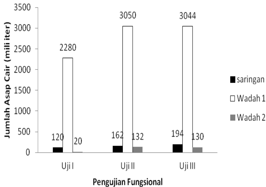
Gambar 8. Hasil asap cair pengujian fungsional
