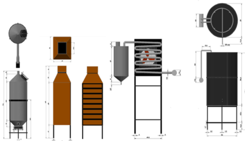
Gambar 2. Gambar rekayasa masing-masing komponen unit penghasil asap cair yang terintegrasi dengan pengering kabinet
