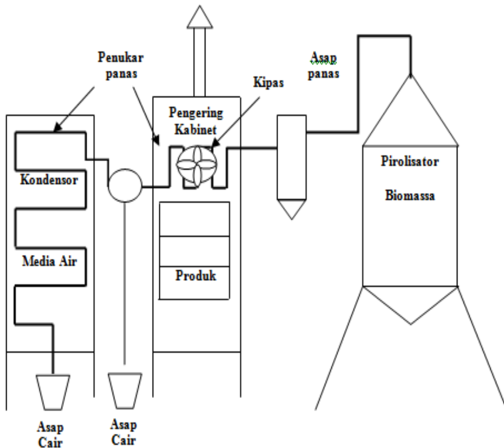
Gambar 1. Skema sistem unit penghasil asap cair dan pengering kabinet
